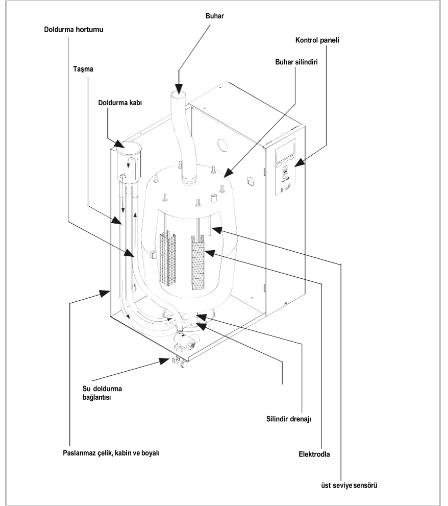
XTP-E Serisi Nemlendirici Parçaları
