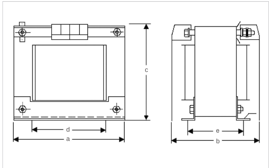
ST Transformatör
