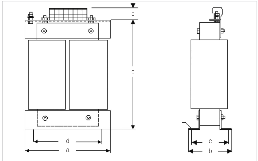
SDS Transformatör
