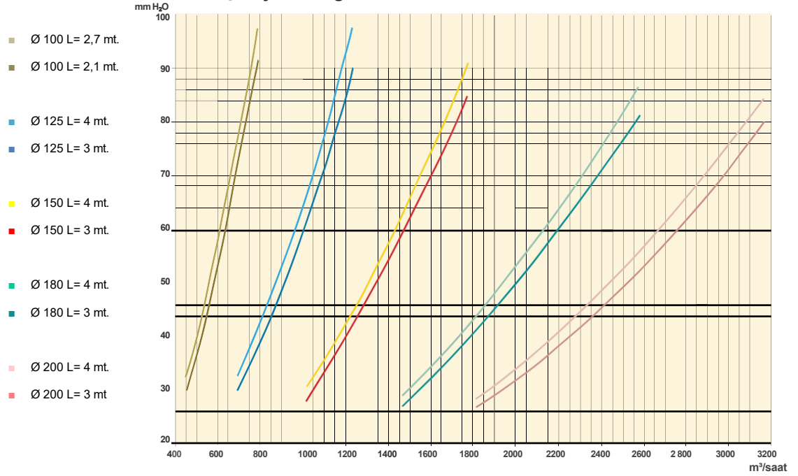
Basınç Kaybı Grafiği
