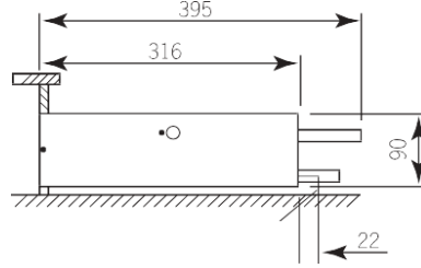
Yandan görünüş
