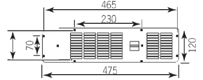
Önden görünüş
