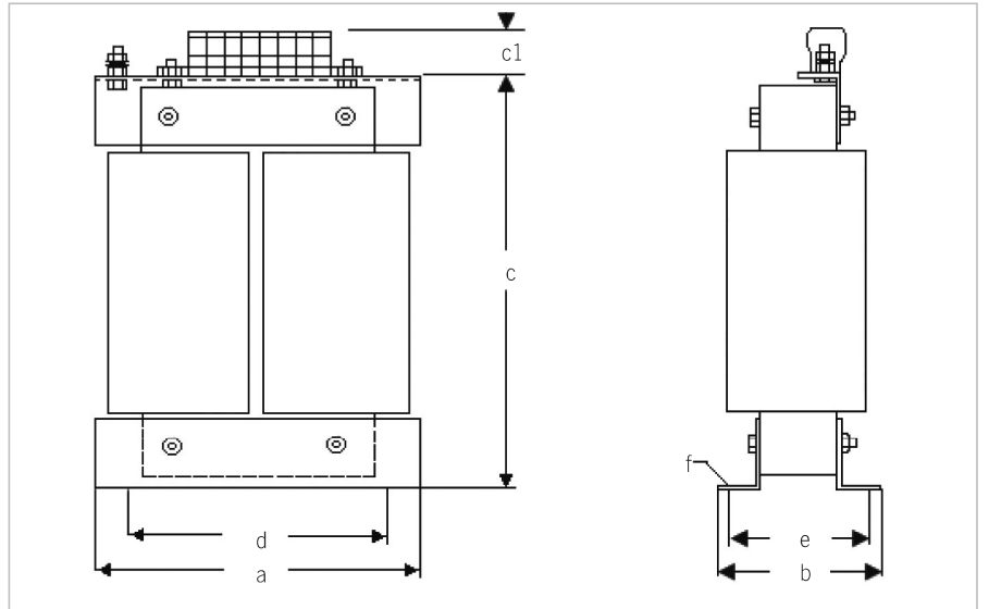
SDS Transformatör
